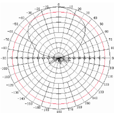
2400MHz E-Plane
