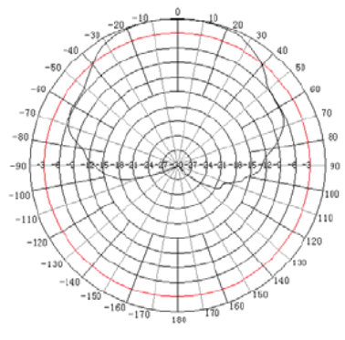
2400MHz H-Plane
