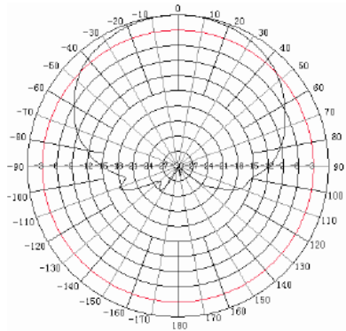
890MHz H-Plane
