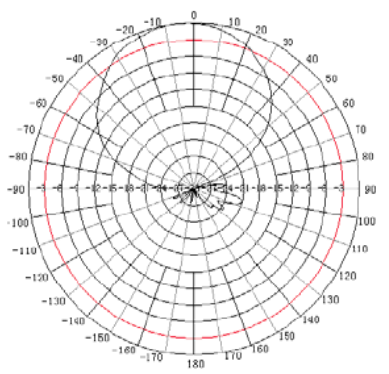
1800MHz E-Plane
