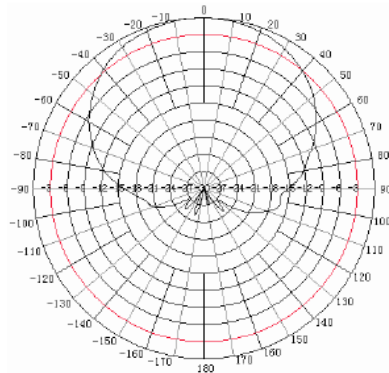
1800MHz H-Plane
