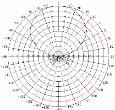
890MHz E-Plane
